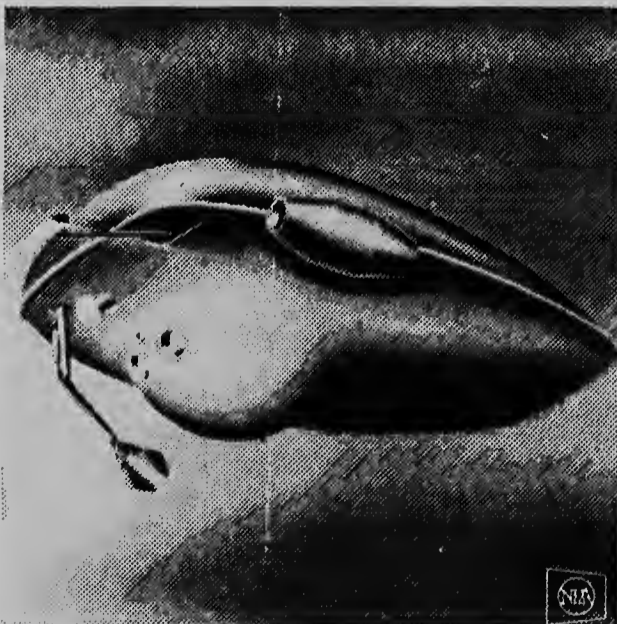
E dibujo aki ta di Aluminat, qu a costa tres millon dollar y por bisa tres homber. Un di nan ta observando boca abao a traves di un di e bentanan di Plexiglas di dies centimeter gureso. E ta pisa 75 tonelada y por laba 4560 meter cu 1359 kilo di instrumentonan cientifico. El a ser construi pa General Dynamics na Groton, Connecticut.
